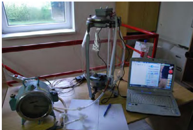
Obr. 6.1 Měřicí zařízení pro ověření reakce O 3 – NH 3
