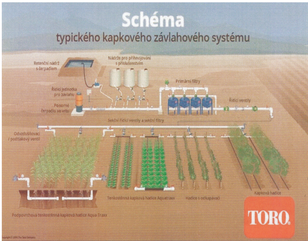
Obr. 18 Schéma možných provedení kapkových závlahových systémů podle firmy TORO
