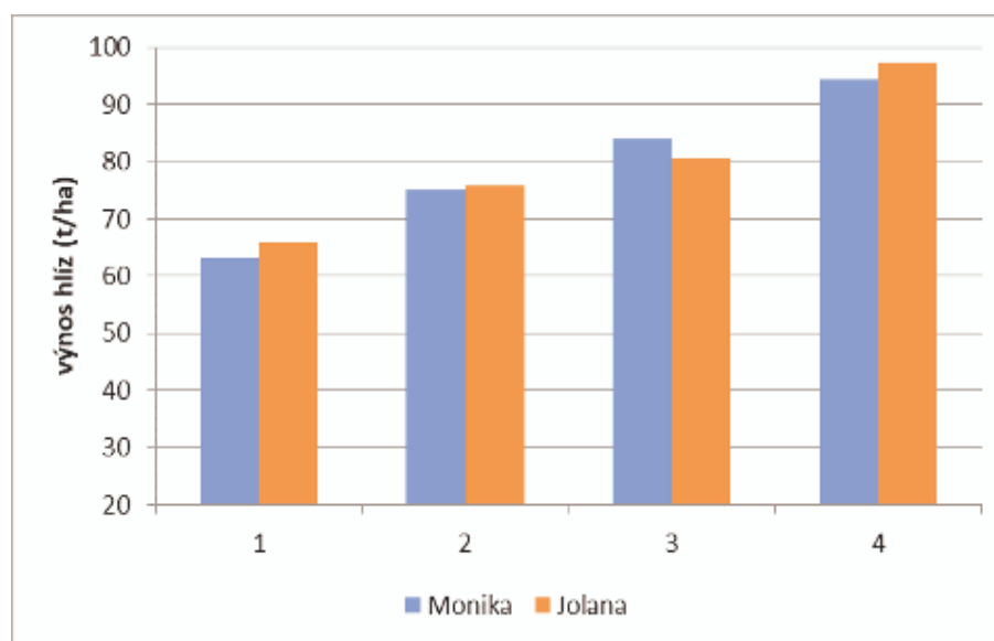
Obr. 5 Vliv variant kapkové závlahy na výnos hlíz v roce 2016
