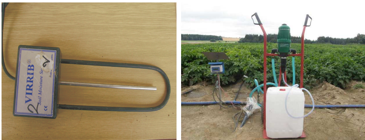
Obr. 4 Čidlo pro řízení závlahy VIRRIB a zařízení pro fertigaci .
