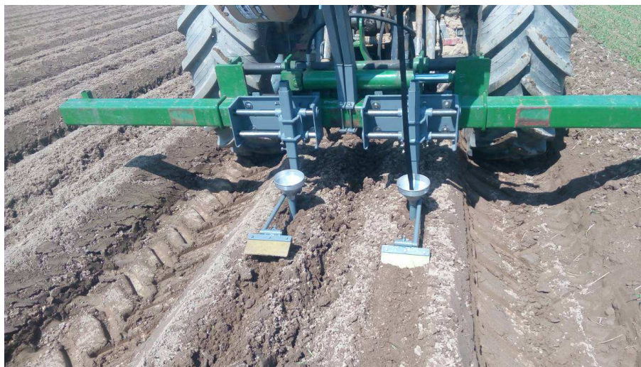
Obr. 21 Ověřování funkčního vzorku zapravovače na pokládání závlahových hadic při polních pokusech
