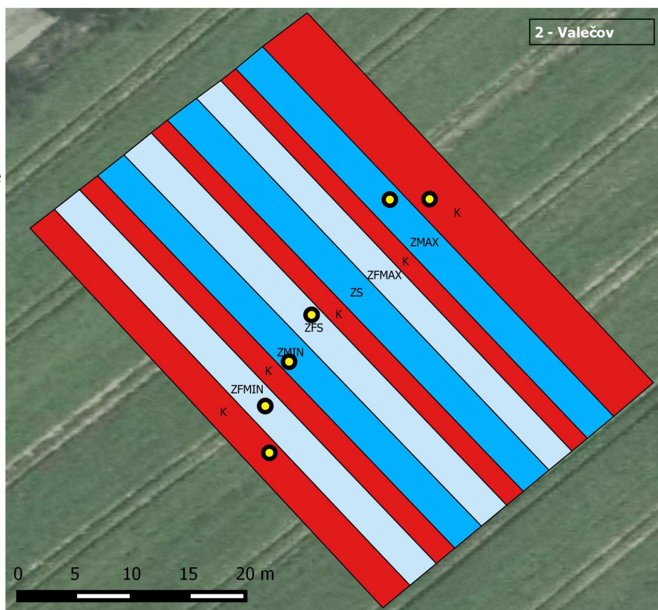
Obr. 2 Schéma pokusné lokality s kapkovou závlahou ve VÚB, s.r.o. H. Brod – Valečov a poloprovozního pokusu Agro Posázaví Okrouhlice – Vadín v r.2016-2018
