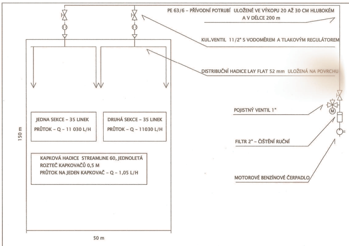
Obr. 3 Schéma instalace kapkové závlahy Agrofim na polním pokusu Okrouhlice – Vadín
