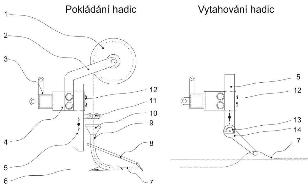
Obr. 20 Schéma konstrukčního návrhu funkčního vzorku zapravovače a vyťahovače kapkových hadic
