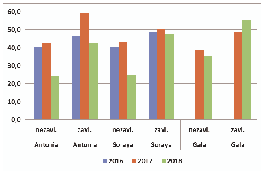
Obr. 25 Porovnání výnosů zavlažovaných a nezavlažovaných brambor v poloprovozním pokusu v letech 2016-2018 (Vadín, t/ha)
