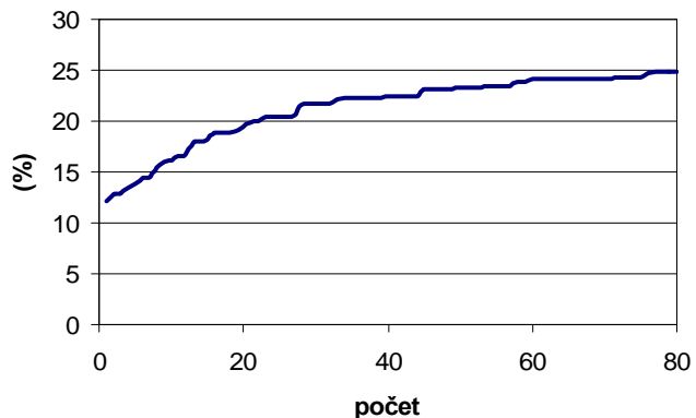
Obr. 5: Průběh rozložení vlhkosti balíků při naskladňování
