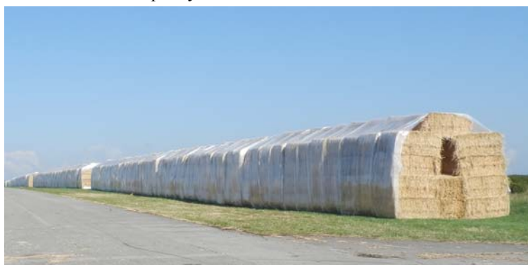
Obr. 1: Technologie uložení a skladování slámy ve stozích obalených smršťovací folií
