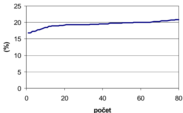
Obr. 6: Průběh rozložení vlhkosti balíků při vyskladňování
