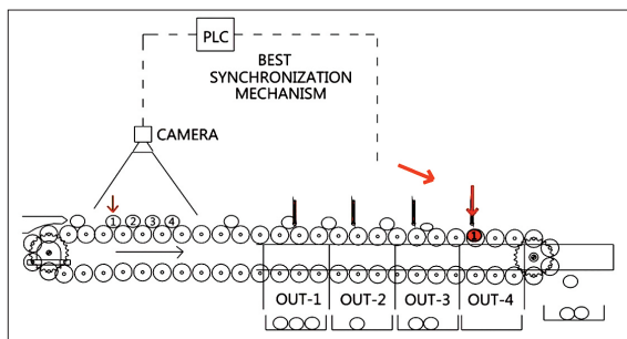
50 Schéma optického třídícího zařízení určeného pro barevné třídění pranych a loupaných brambor
