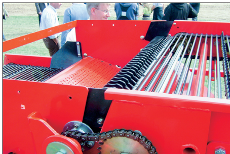
30 Vzduchový oddělovač příměsí u sklízeců nahrazuje mechanická zařízení pro oddělování hlíz a příměsí
