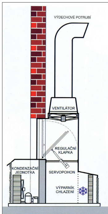
46 Schéma integrované směšovací komory pro úpravu klimatu ve skladu
