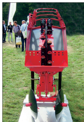
17 Nové technické řešení pásového sázečího ústrojí nepoškozuje sadbu
