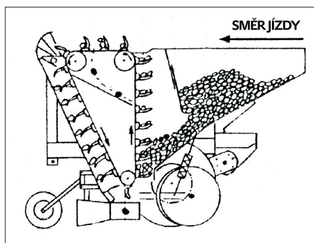
20 Inovace sázecího ústrojí naklopením a novým tvarem vysazovacích pohárků s elektronickým řízením pro zvýšení přesnosti sázení
