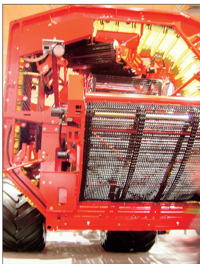
33 Nový typ vynášecího dopravníku sklízecí s kapsami z polyuretanu pro dodatečné intenzivní prosévání půdy šetrné k hlízám
