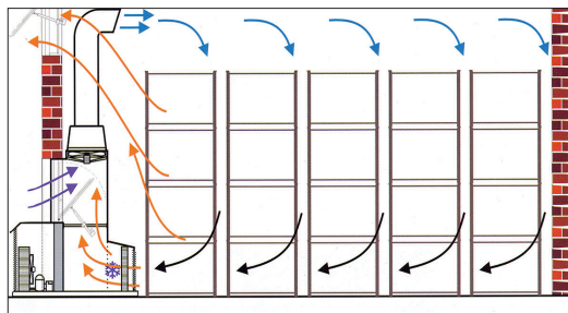
39 Schéma průchodu větracího vzduchu v paletovém skladu brambor
