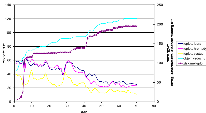
Obr. 2: Graficky znázorněné výsledky pokusu s jímáním tepla z kompostovacího procesu
