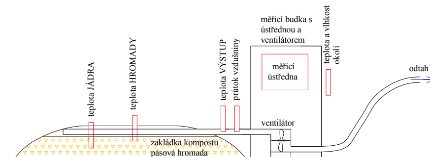
Obr. 1: Schéma měření
