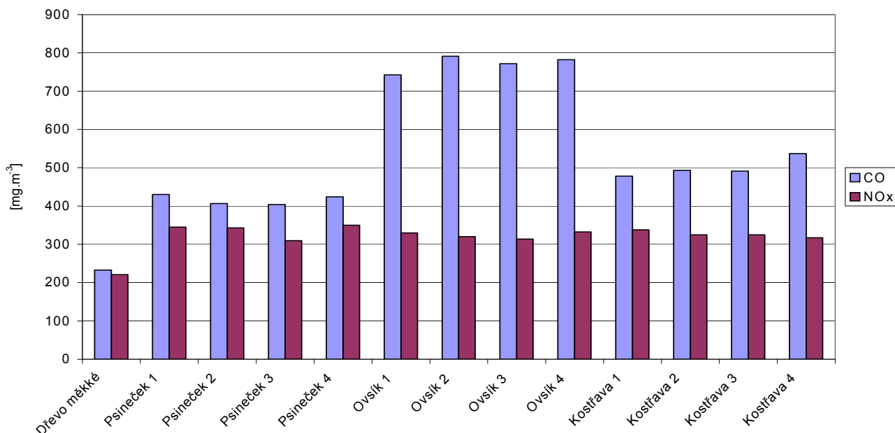
Obr. 8: Půlhodinové průměry emisí CO a NO x pro různá paliva u kotle V25
