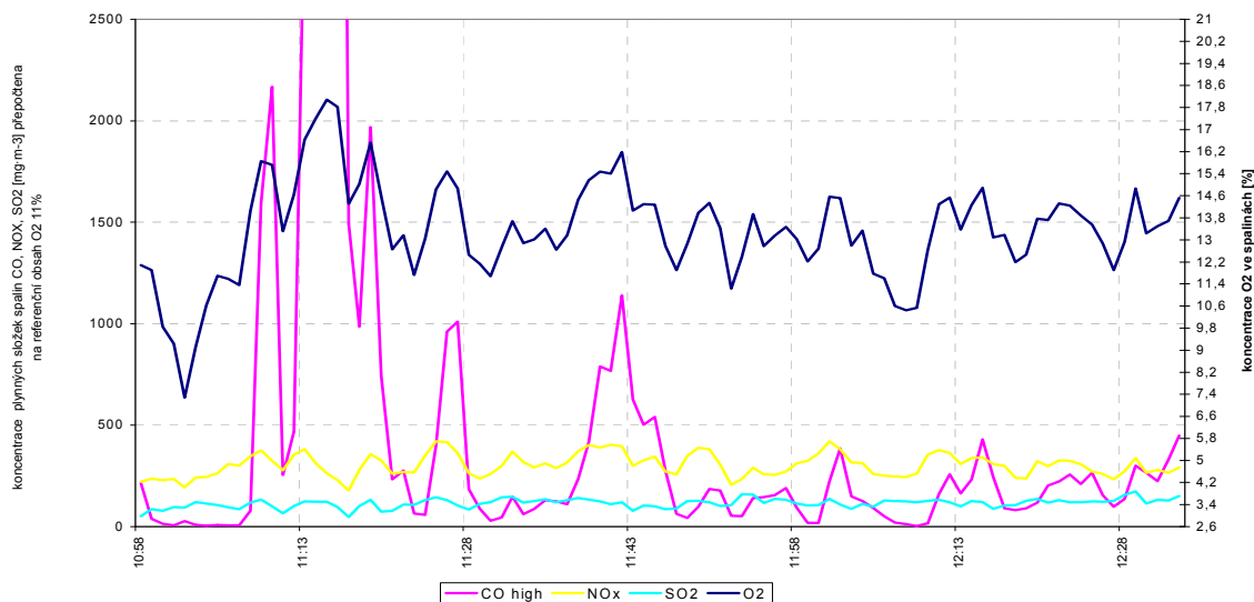
Obr. 4: Průběh koncentrací O 2 , CO, NO x a SO 2 při spalování psinečku
