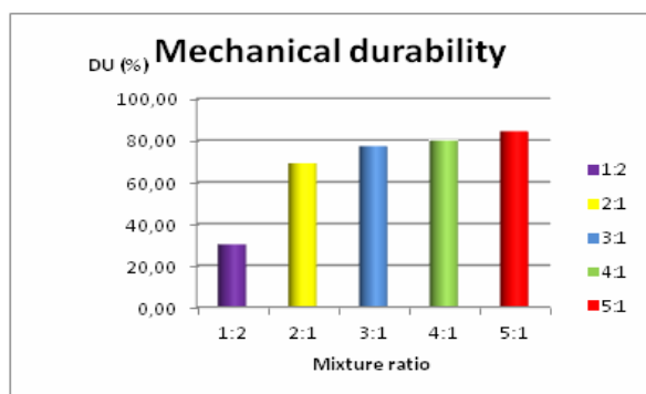
Graf 1: Mechanická odolnost briket odpadní konopné biomasy Mechanical durability of briquettes made of hemp waste biomass
