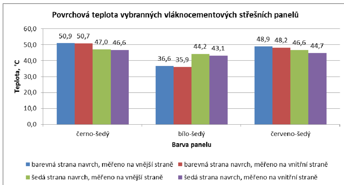
Obr. 18 Vliv barevného provedení cemento vláknitých panelů na teploty jejich povrchu
