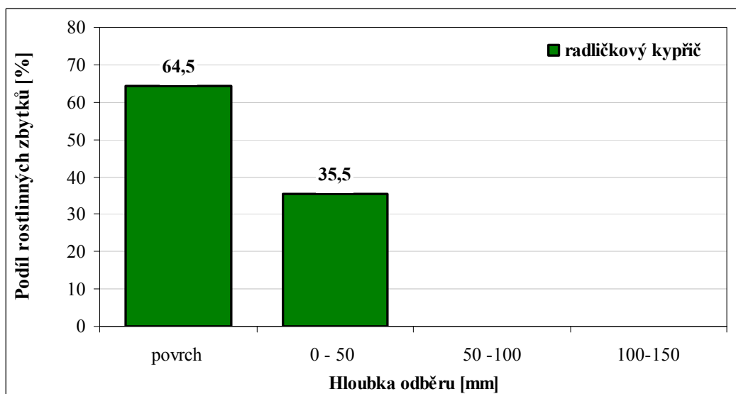
Obr 9 Rozmístění posklizňových zbytků ve zpracovávaném profilu půdy po zpracování radličkovým kypřičem s podřezávacími radličkami
