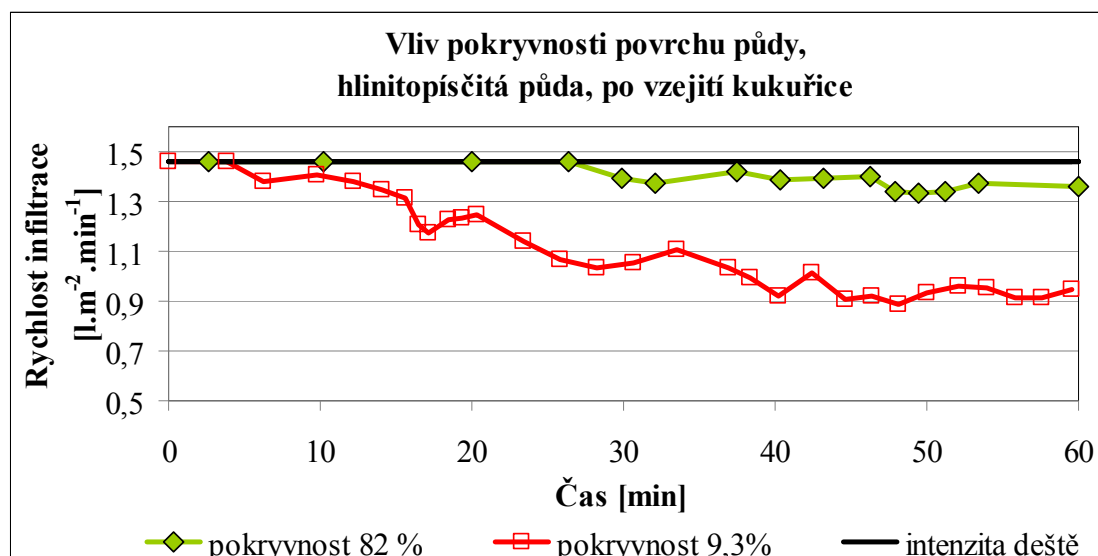
Obr. 12 Porovnání vsakující vody při dešťové srážce s konstantní intenzitou 1,46 \text{ mm}\cdot\text{min}^{-1} ( 87 \text{ mm}\cdot\text{h}^{-1} ) po dobu 60 min na pozemku se vzešlou kukuřicí; písčitohlinitá půda
