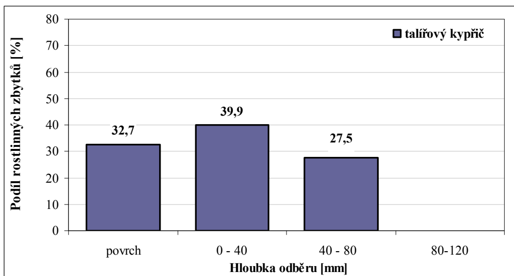
Obr. 8 Rozmístění posklizňových zbytků ve zpracovávaném profilu půdy po zpracování talířovým kypřičem (odhad výnosu slámy na hodnoceném stanovišti 5,3 \text{ t} \cdot \text{ha}^{-1} )
