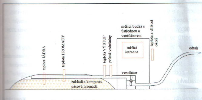
Obr. 1 – Schéma měření
